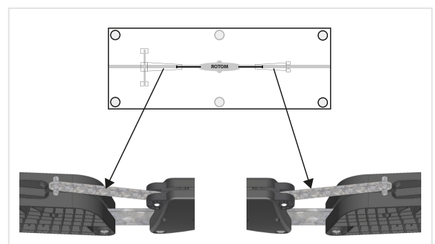
Metallzughebel ausgekoppelt (keine Funktion)
