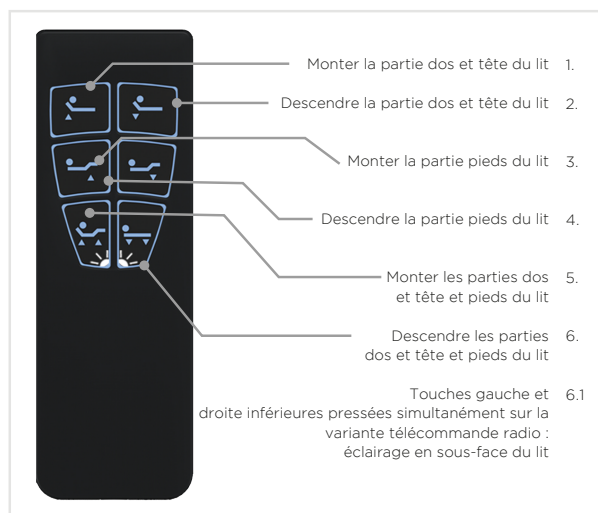
télécommande 2M RF
